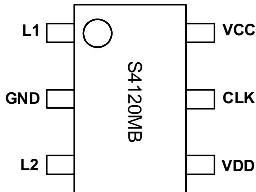
图 12 管脚封装图
